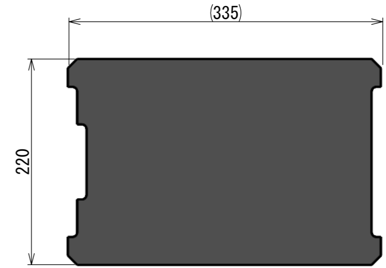
フタ側クッション材 1:4
